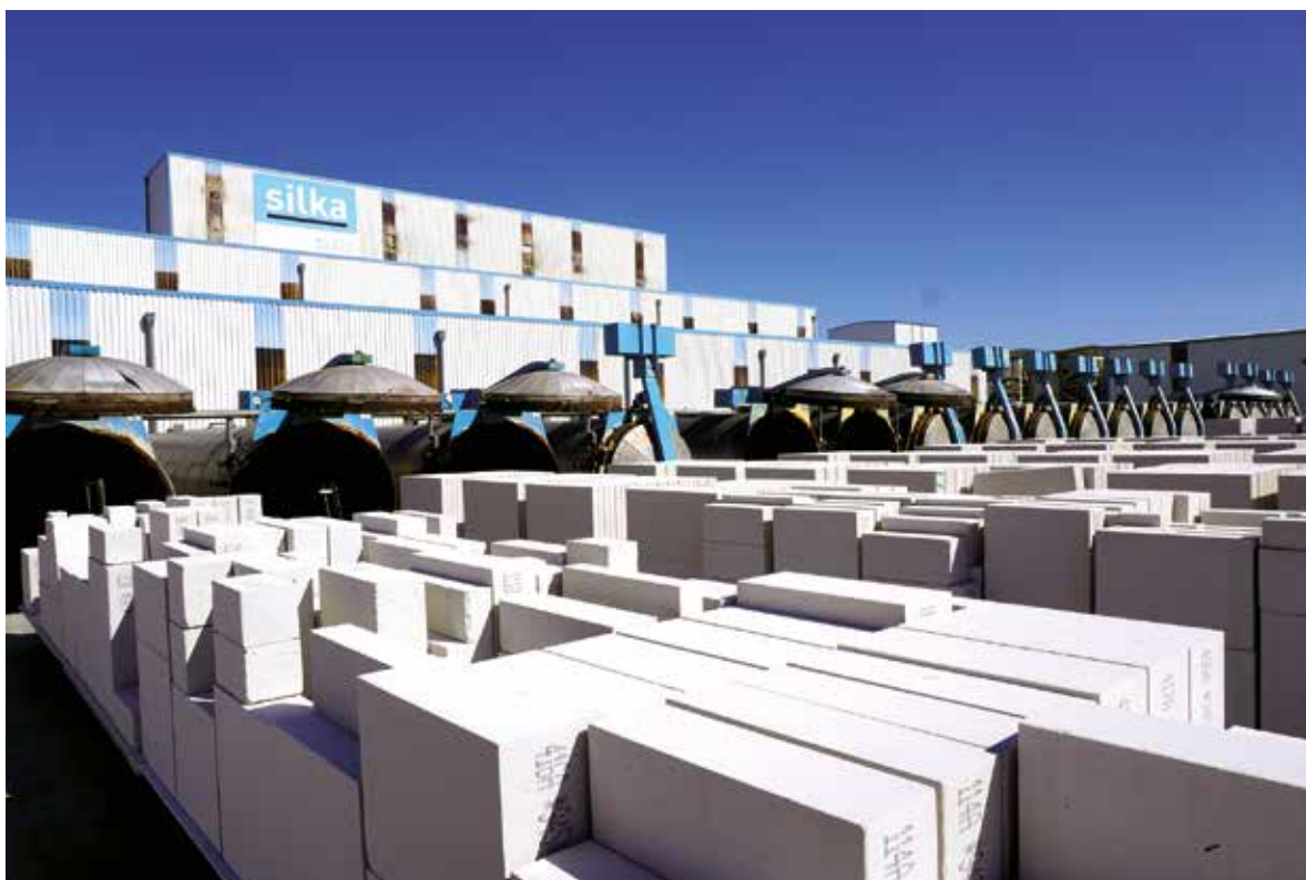
Vor den geöffneten Dampfdruckkesseln, den Autoklaven, kühlen die gehärteten Kalksandsteine ab und warten auf ihre Verladung, Foto: BGR.
